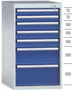
Schubladenschrank SEB1000-07EP-001
